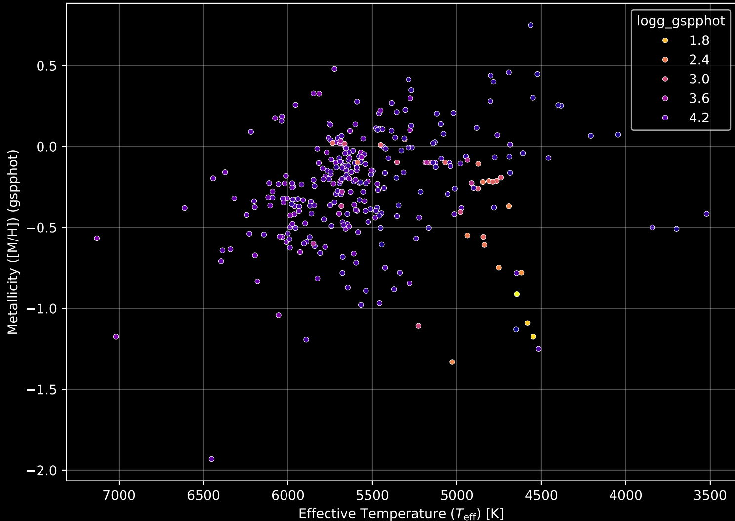
GALAH DR4 Field: [7012] Stellar Population Parameters (n= 303)
