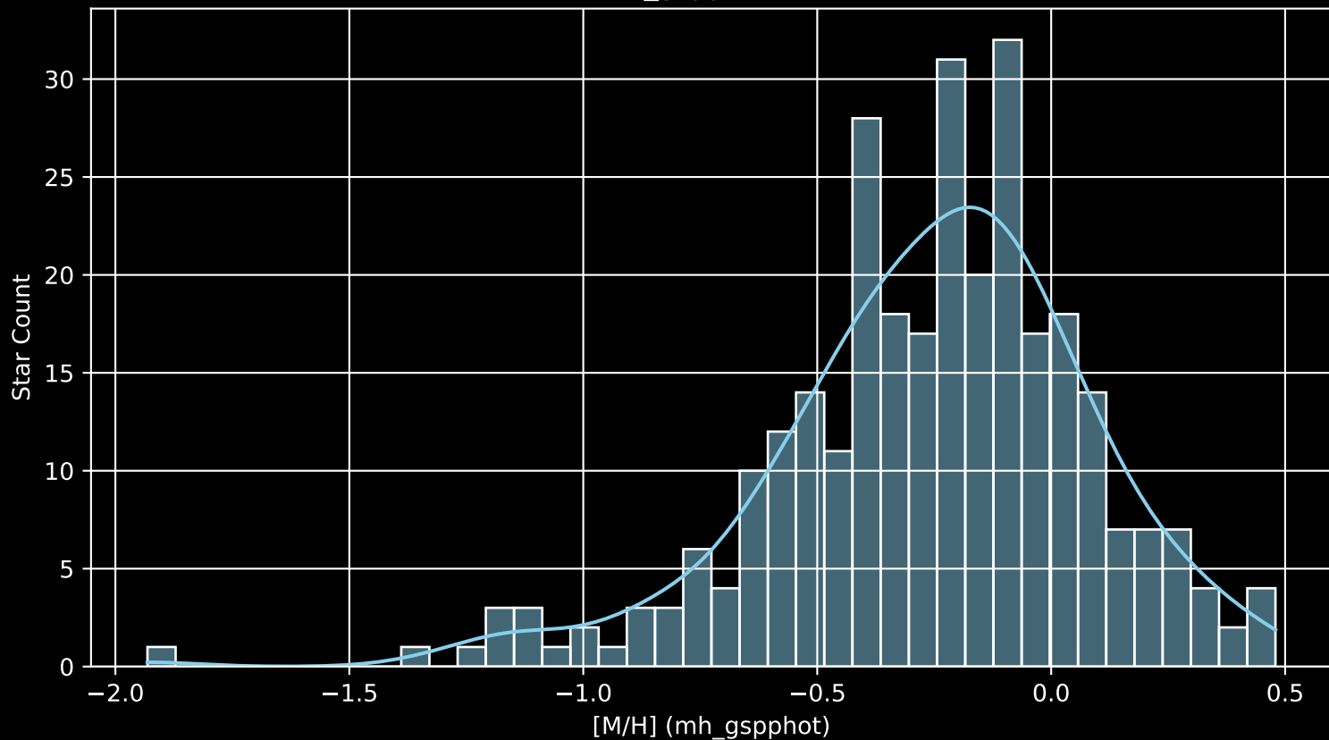
GALAH DR4 Field: [7012] [M/H] (mh_gspphot) (n= 302)
