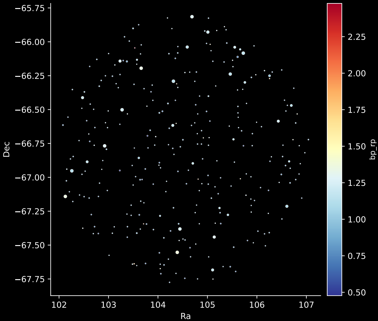
GALAH DR4 Field: [7012] Stars: 303
